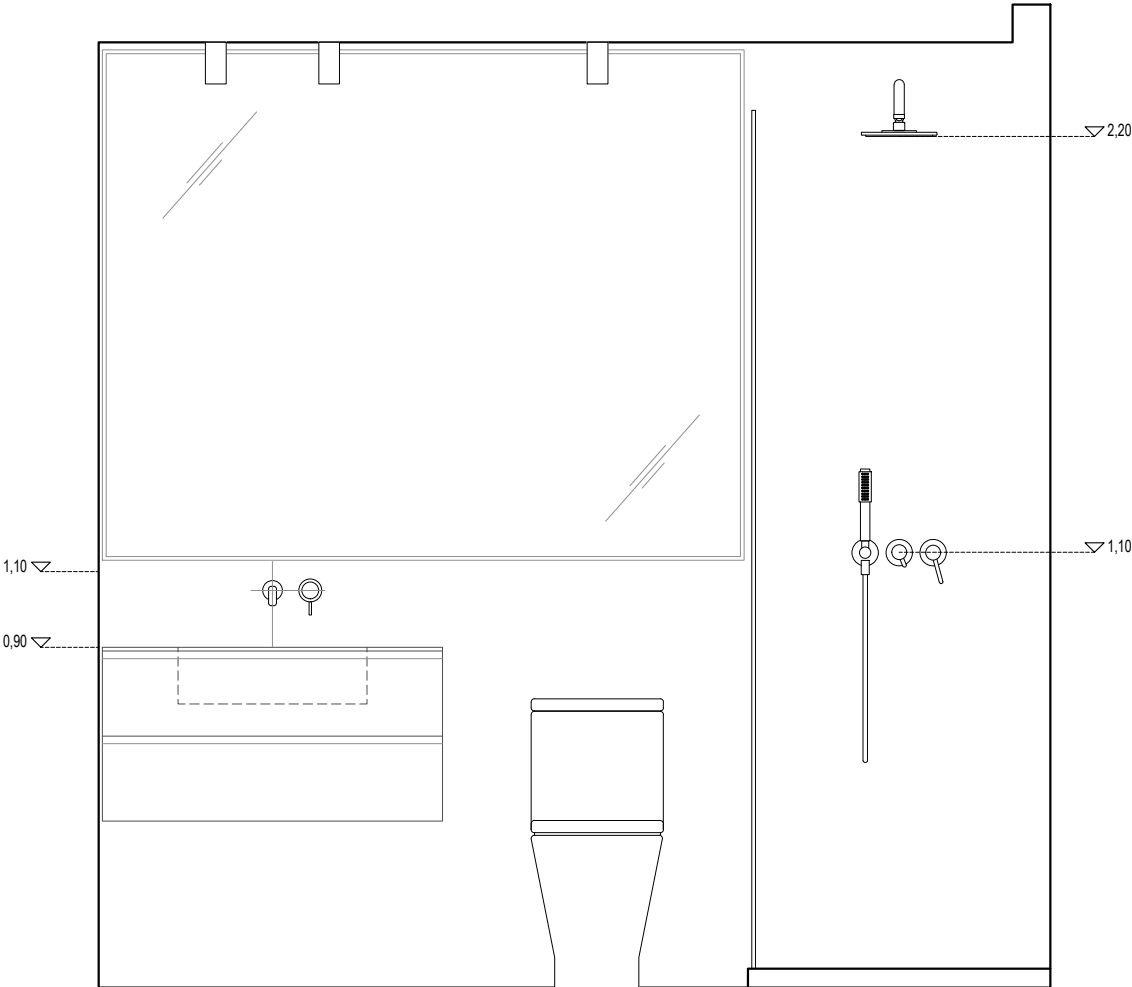
ALÇAT B-B'
