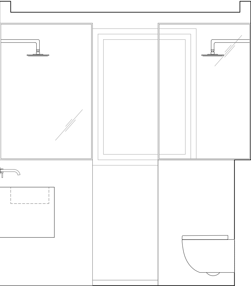
ALÇAT A-A'
