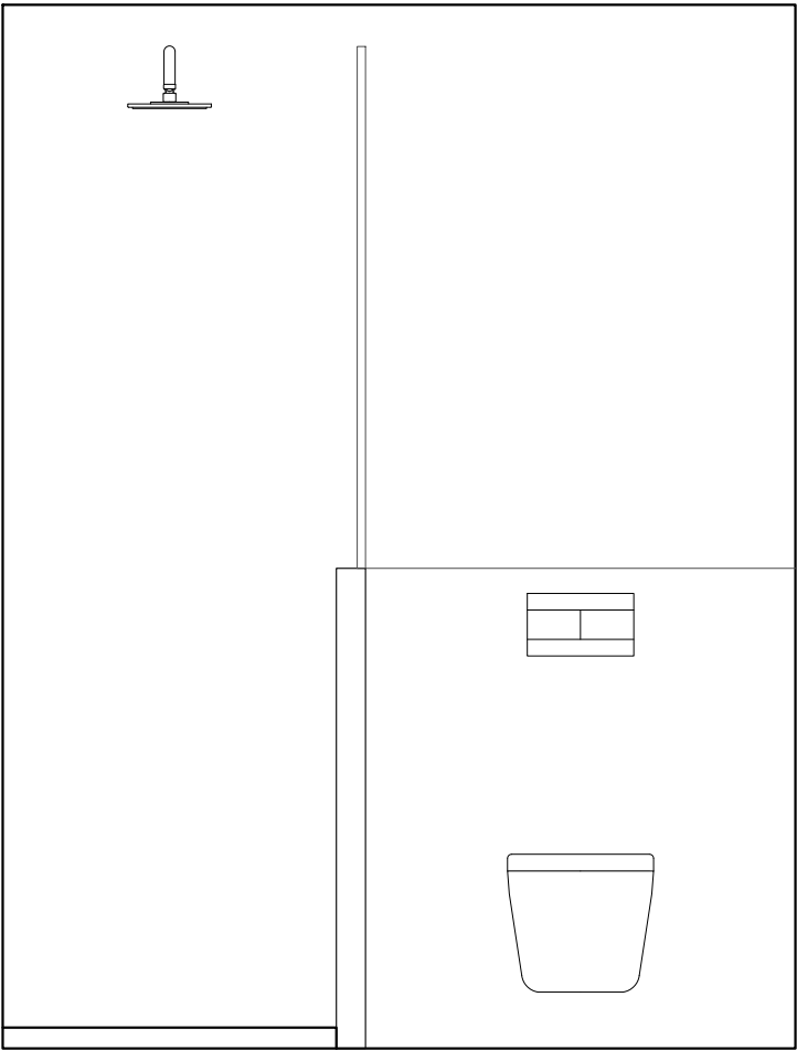
ALÇAT C-C'
