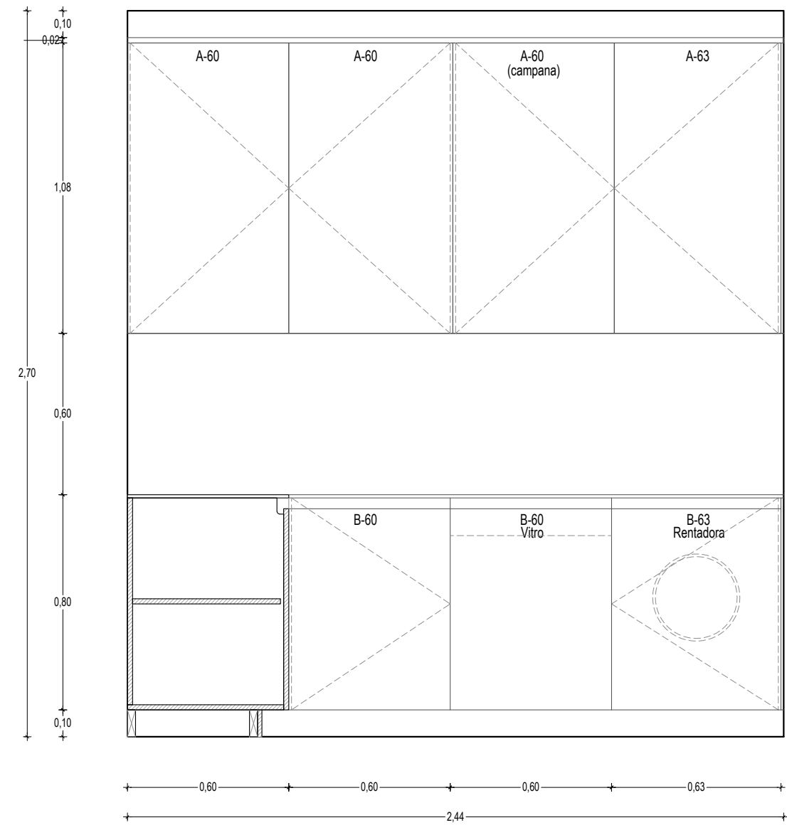
ALÇAT C-C'
