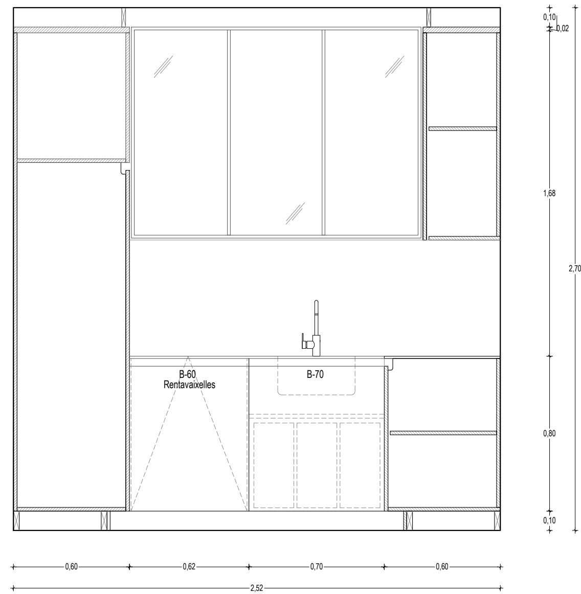
ALÇAT B-B'
